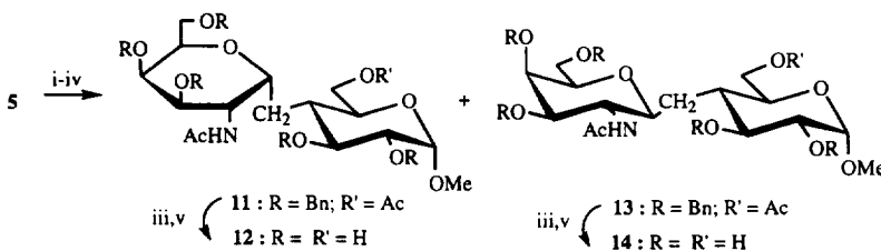
Scheme 5. Reagents: i) \text{Bu}_3\text{SnH} , AIBN, toluene; ii) \text{HCl} , \text{MeOH} ; iii) \text{MeONa} , \text{MeOH} ; iv) \text{Ac}_2\text{O} , \text{pyr} ; v) \text{H}_2 , 10% \text{Pd/C} , \text{MeOH} .
