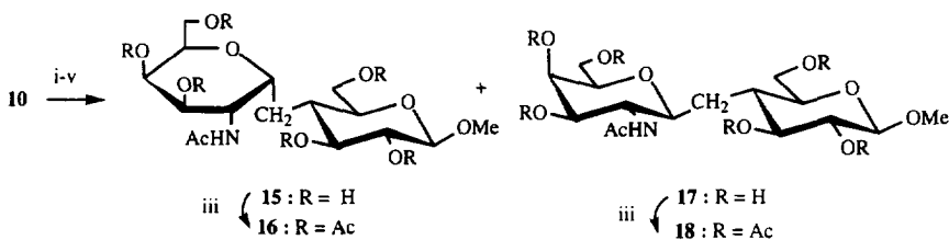
Scheme 6. Reagents: i) \text{Bu}_3\text{SnH} , AIBN, toluene; ii) \text{LiAlH}_4 , THF, 0^\circ\text{C} ; iii) \text{Ac}_2\text{O} , Pyr; iv) \text{MeONa} , \text{MeOH} ; v) \text{H}_2 , 10% \text{Pd/C} , \text{MeOH} .
